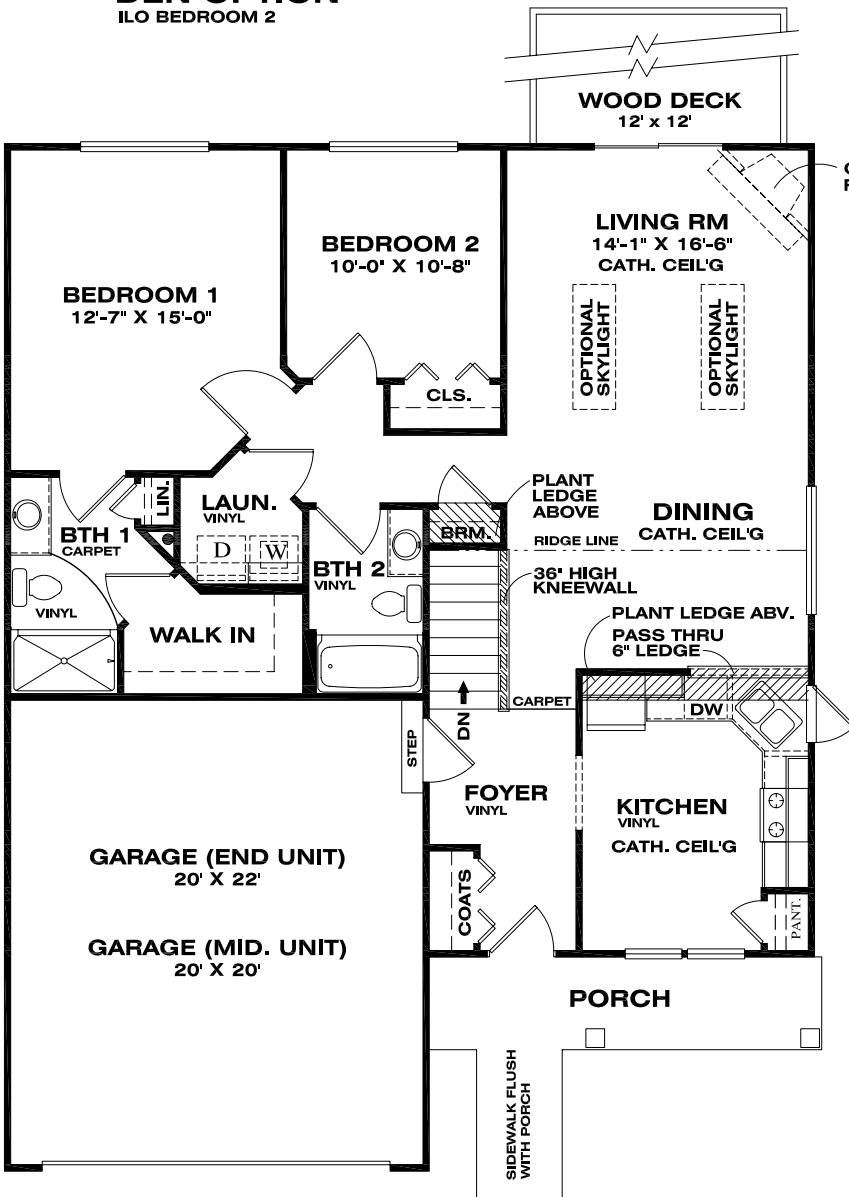
DEN OPTION ILO BEDROOM 2
